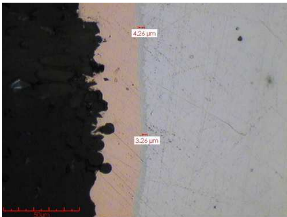
Schliff 1: Detailansicht der Lötstelle mit Vermessung der IZ und Bemerkungen
